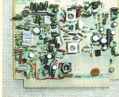
De FM-module voor de Yaesu FT-901.
